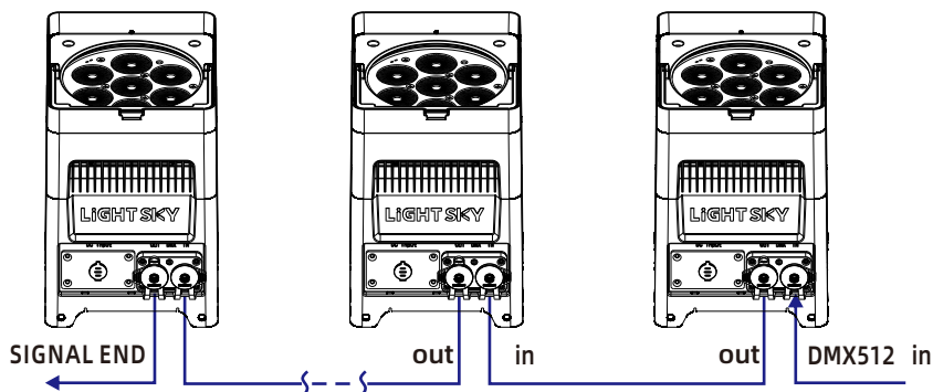
DMX-input
