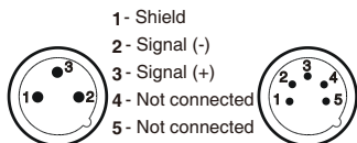
DMX-input
