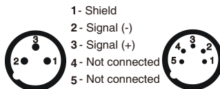
DMX - output
