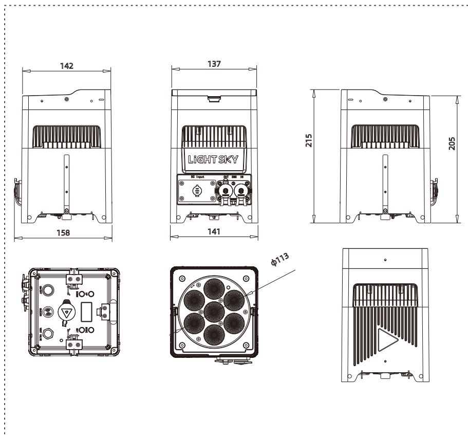
Size-Fig.2 (Unit:mm)
